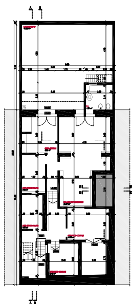
PLANTA PISO -2 SUB-CAVE, ÁREA BRUTA DO PISO (113,02 m²)
