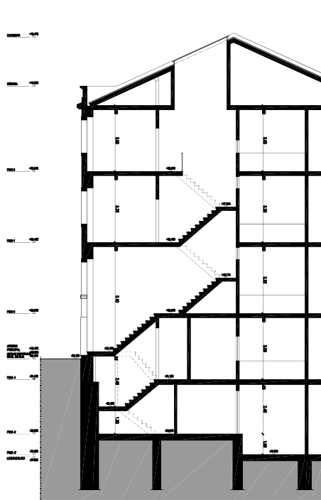
CORTE AA
