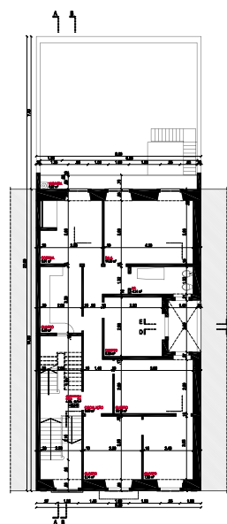
PLANTA PISO 1, ÁREA BRUTA DO PISO (102,08 m²)
