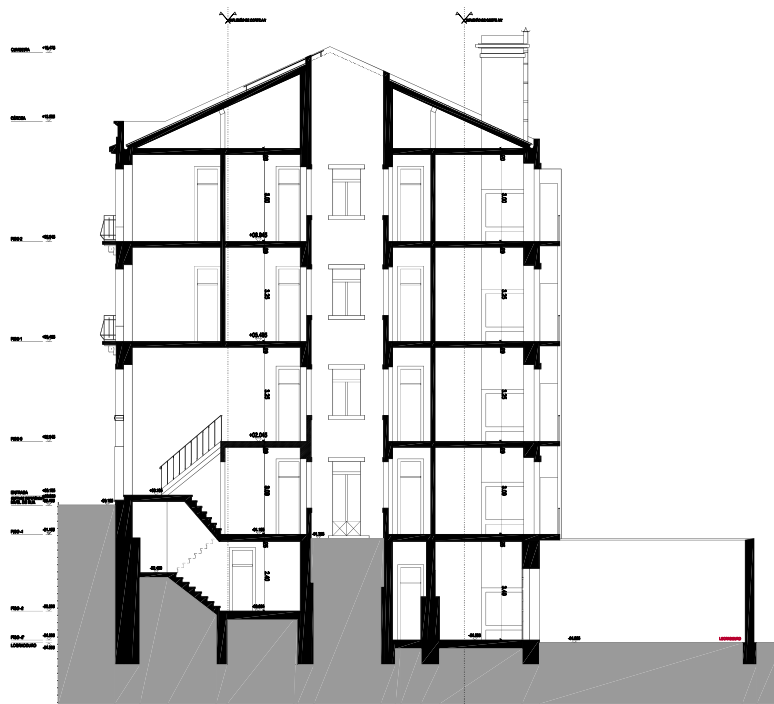
CORTE BB
