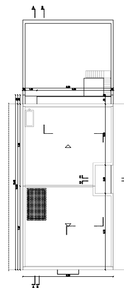
PLANTA COBERTURAS
