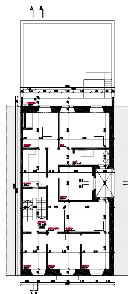
PLANTA PISO 1, ÁREA BRUTA DO PISO (113,34 m²)
