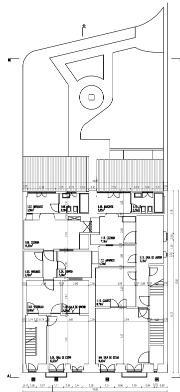
PLANTA PISO 1 ESC. 1:100
