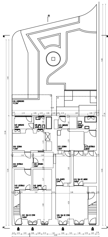
PLANTA PISO 0 ESC. 1:100
