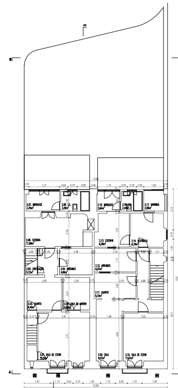
PLANTA PISO 2 ESC. 1:100
