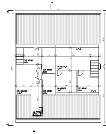
PLANTA PISO 3 ESC. 1:100
