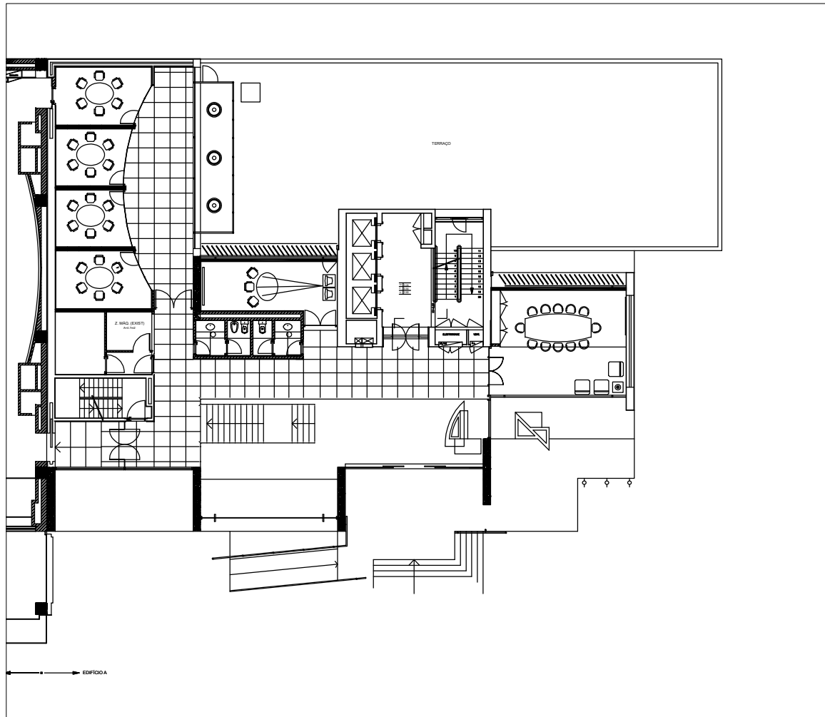
PLANTA PISO 1 ESC. 1:200
