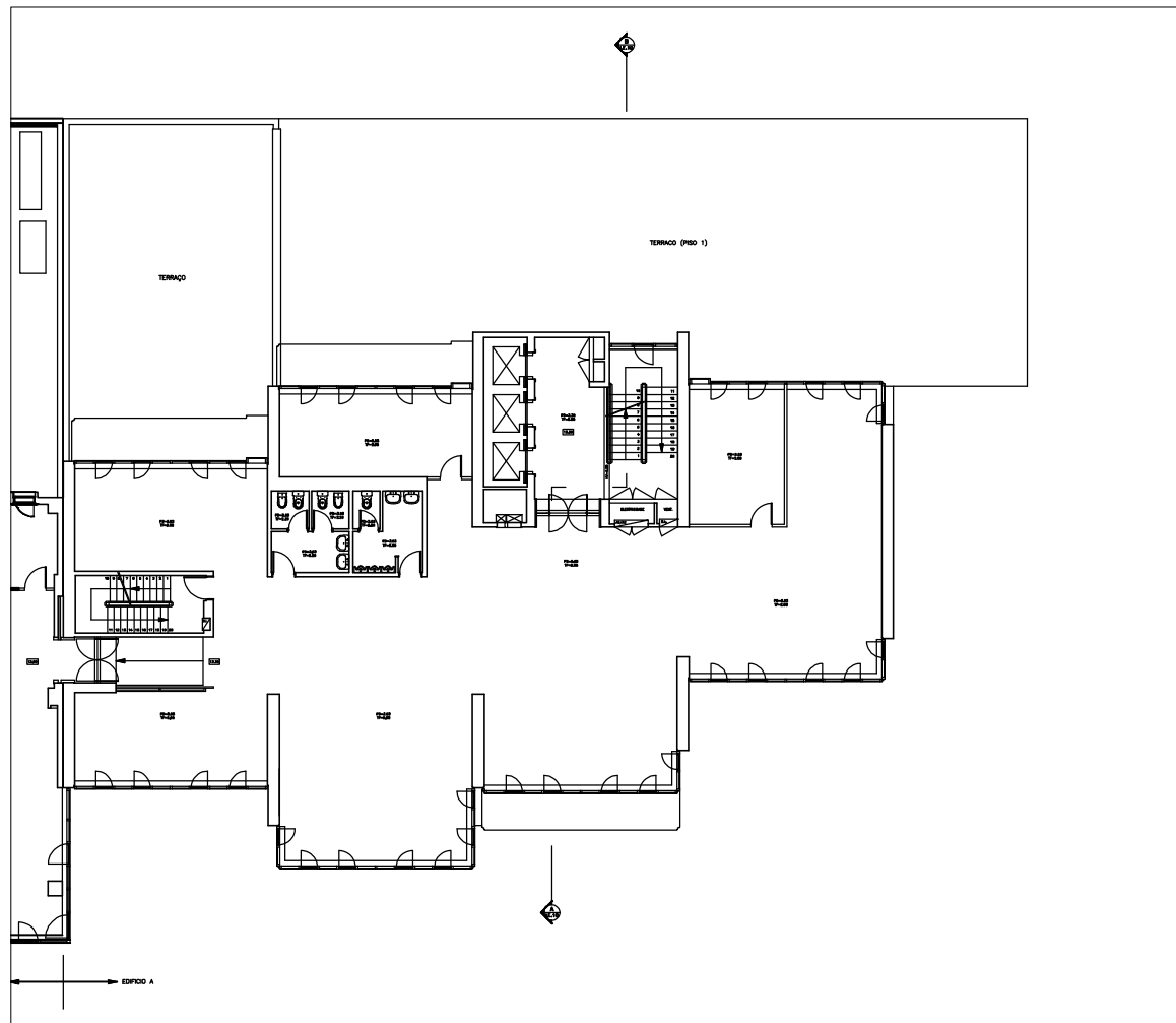
PLANTA PISO 4 ESC. 1:200
