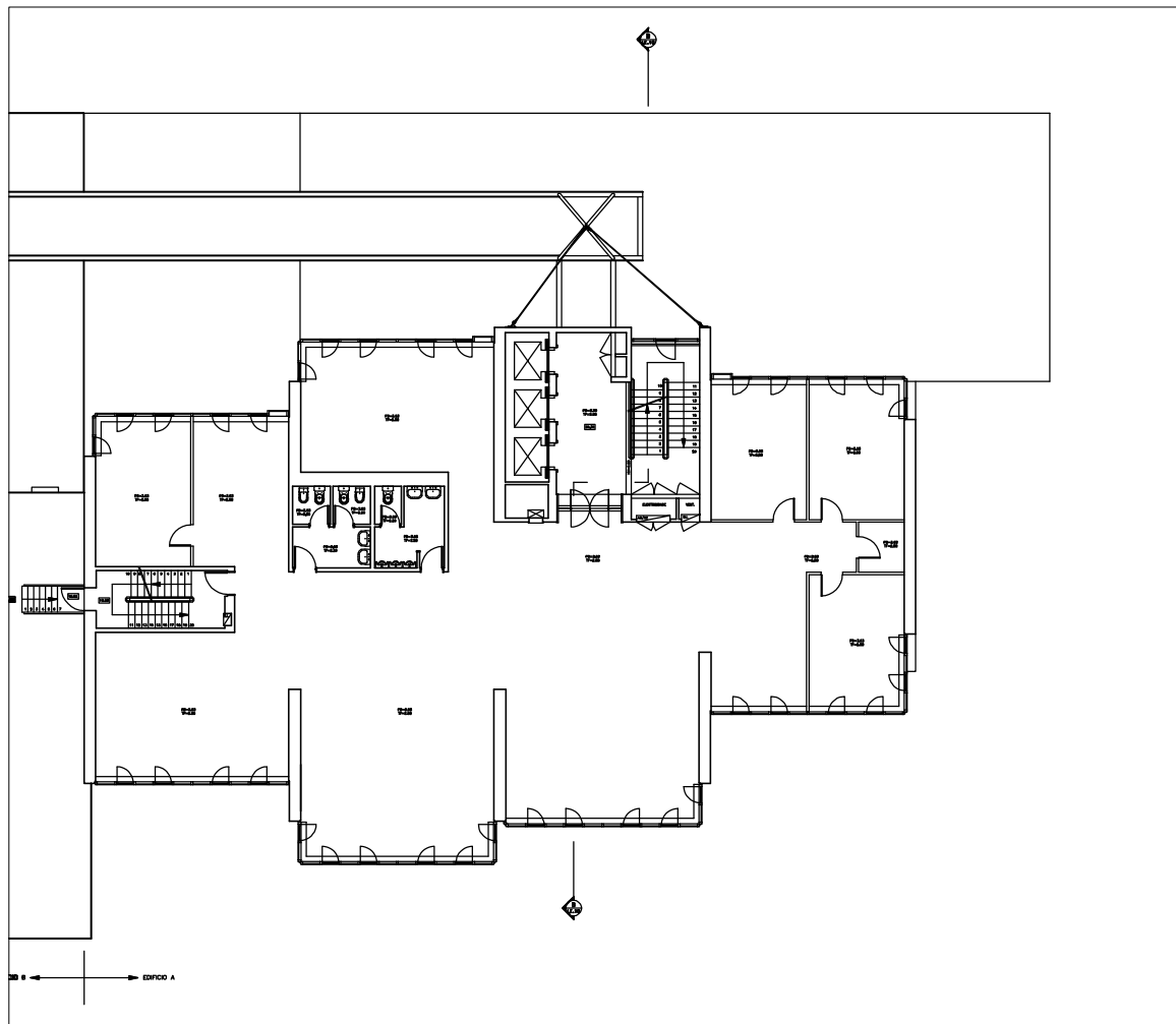
PLANTA PISO 6 ESC. 1:200
