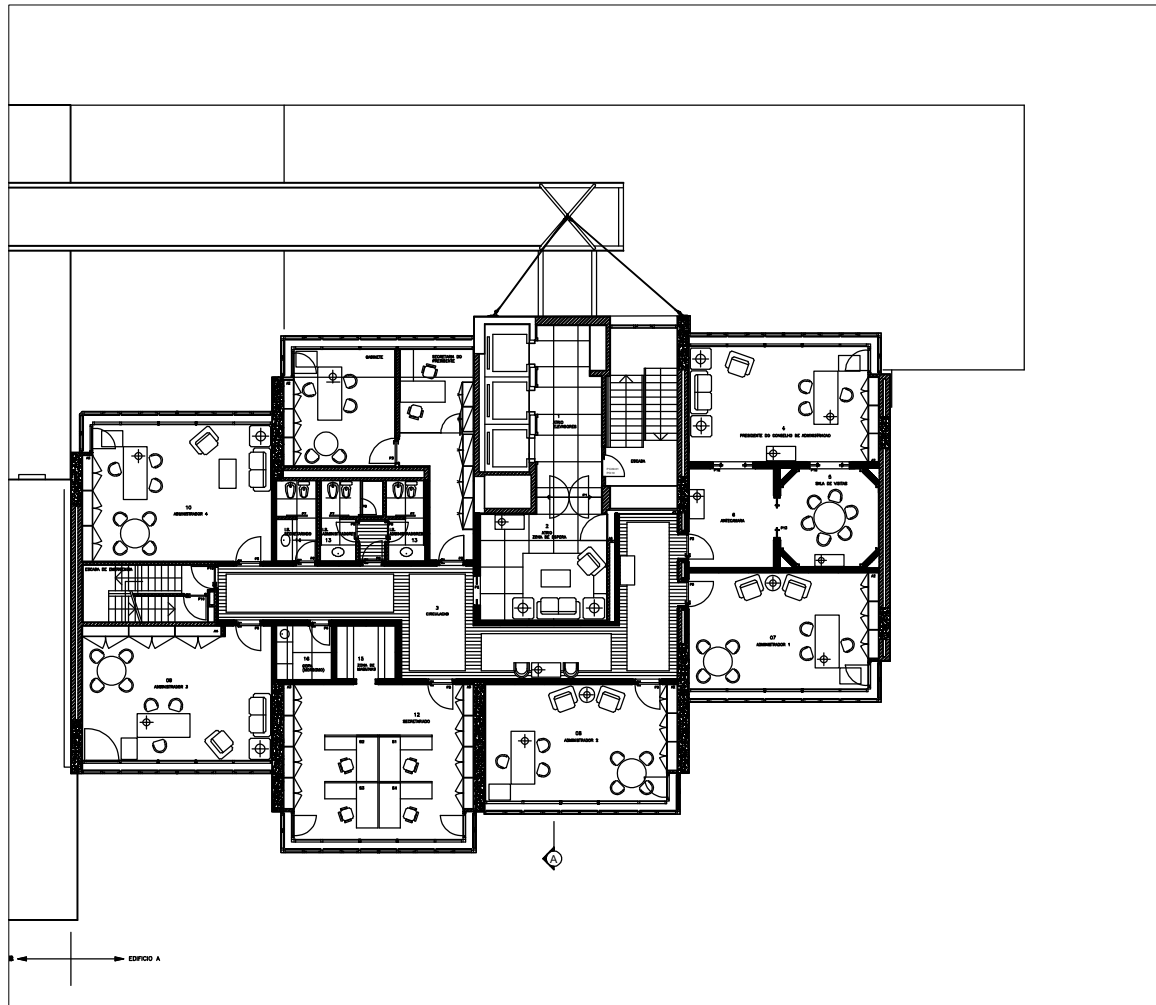
PLANTA PISO 9 ESC. 1:200
