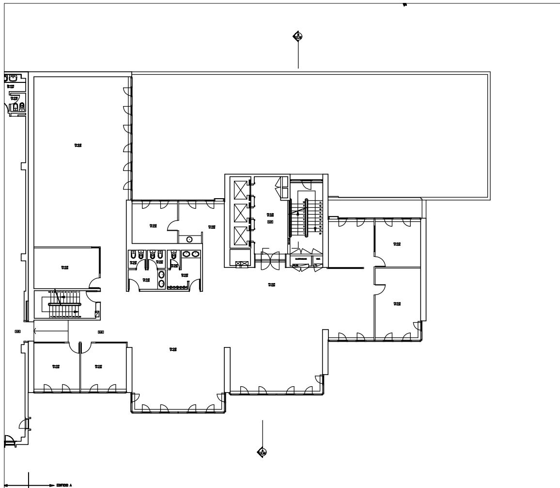
PLANTA PISO 2 ESC. 1:200
