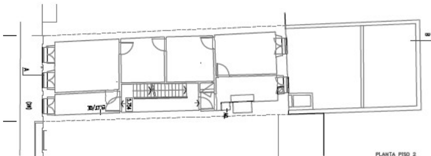
PLANTA PISO 2
